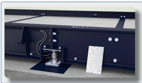
■ La báscula BPBSH de gran capacidad con células de compresión modelo GIP.
