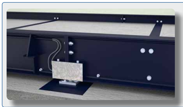
■ Unión de las vigas y las traveseras, mediante tornillería zincada de calidad 8.8.
